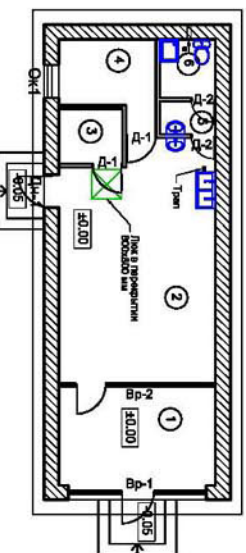
ПЛАНИ ПОМЕЩЕНИЙ М 1:100
